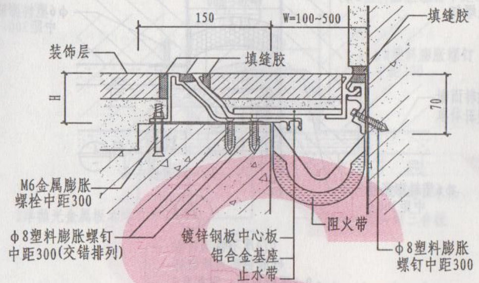
① 楼、地面与墙面胶条防震型
