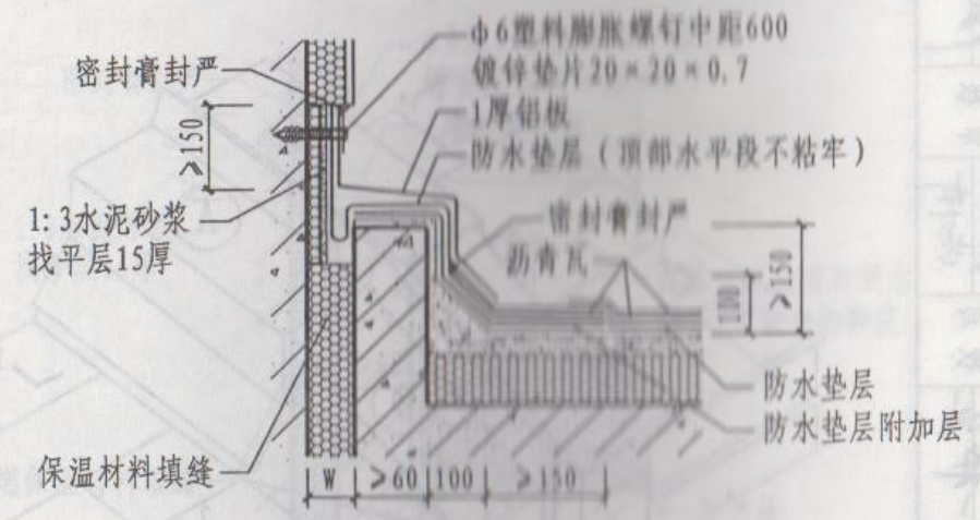
2 高低跨变形缝
