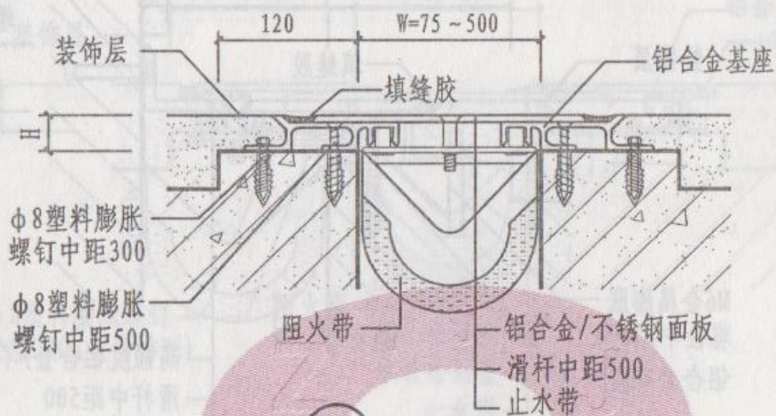
① 楼、地面金属盖板嵌平型
