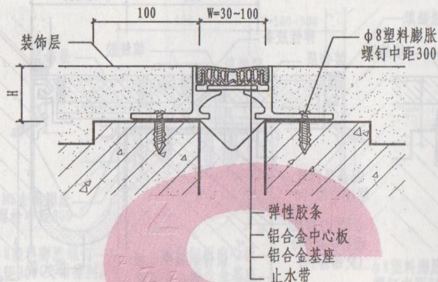
① 楼、地面单列嵌平胶条型
