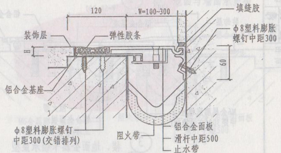
④ 楼、地面与墙面双列嵌平胶条型
