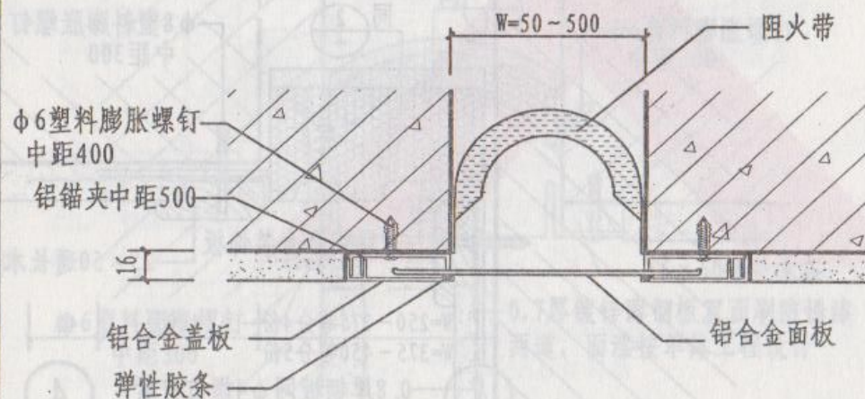
③ 内墙、顶棚双列金属卡锁型
