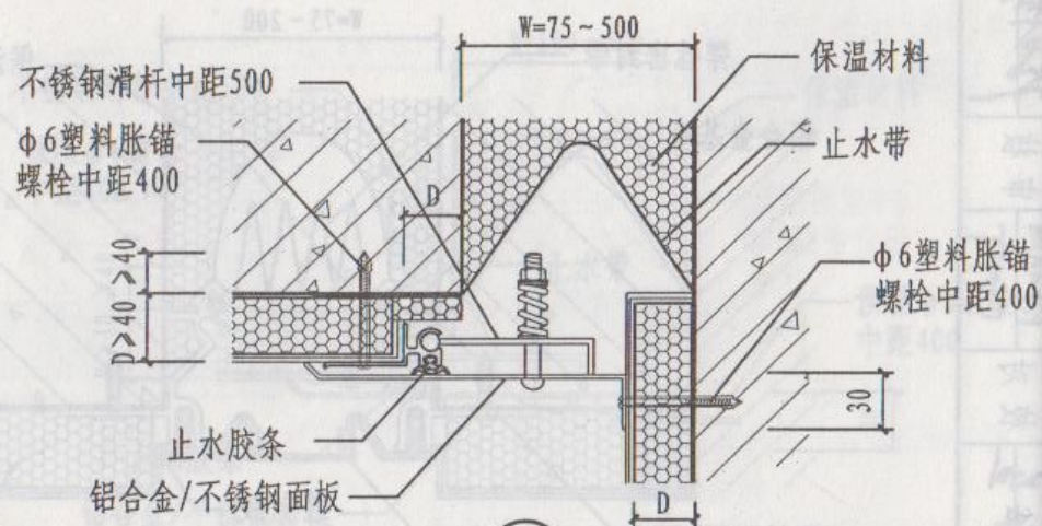
② 外墙与墙盖板防震型
