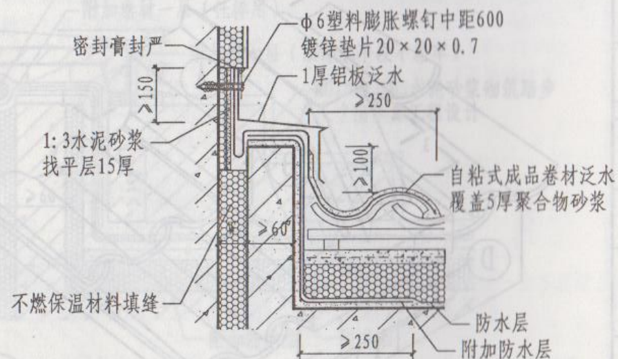
③ 高低跨变形缝
