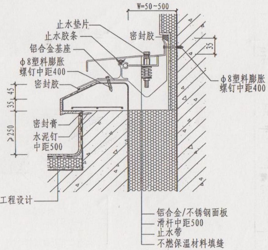
② 屋面与墙面金属盖板防震型
