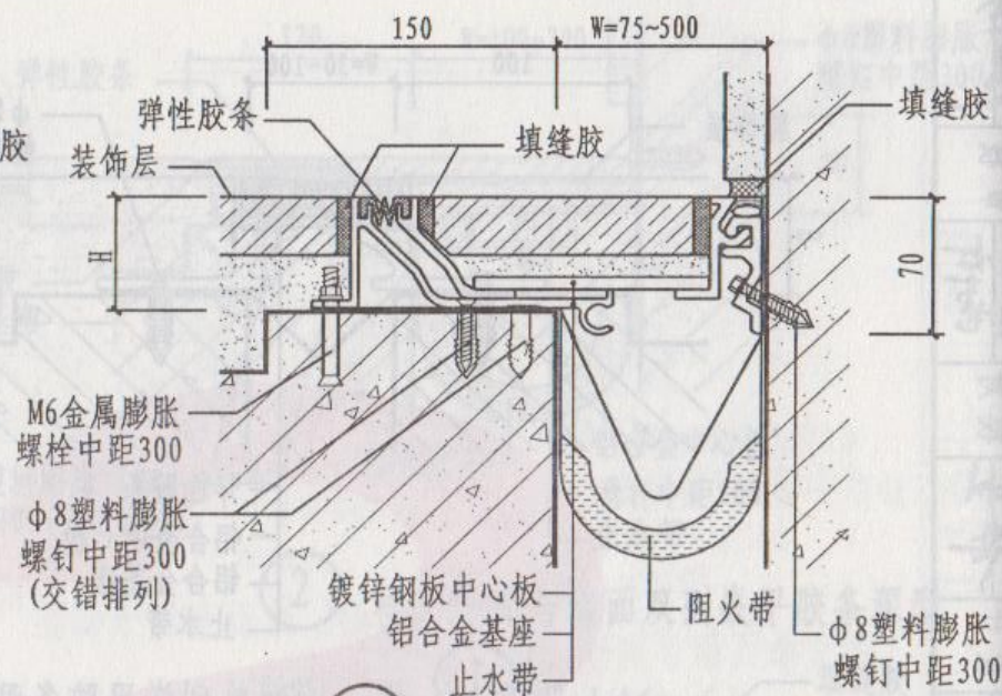
② 楼、地面与墙面双列防震型
