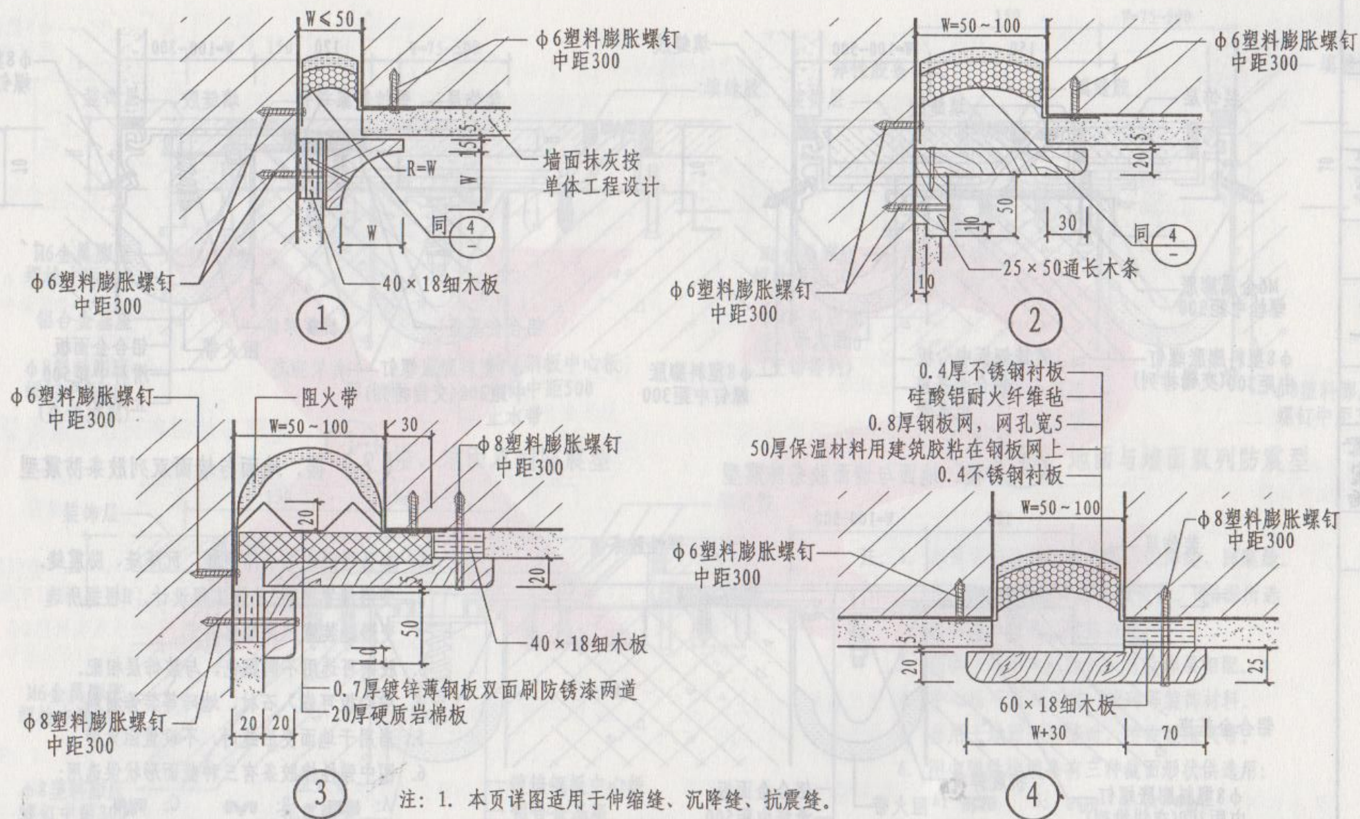
内墙变形缝(一)
