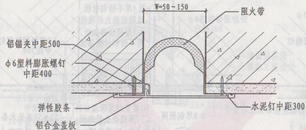
① 内墙、顶棚单列金属卡锁型
