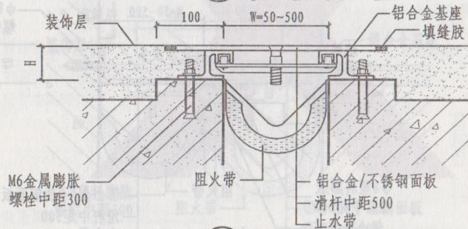
③ 楼、地面承重 II 型
