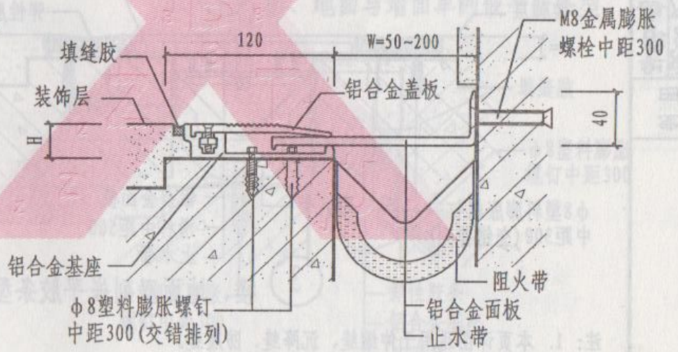
④ 楼、地面与墙面金属卡锁承重型
