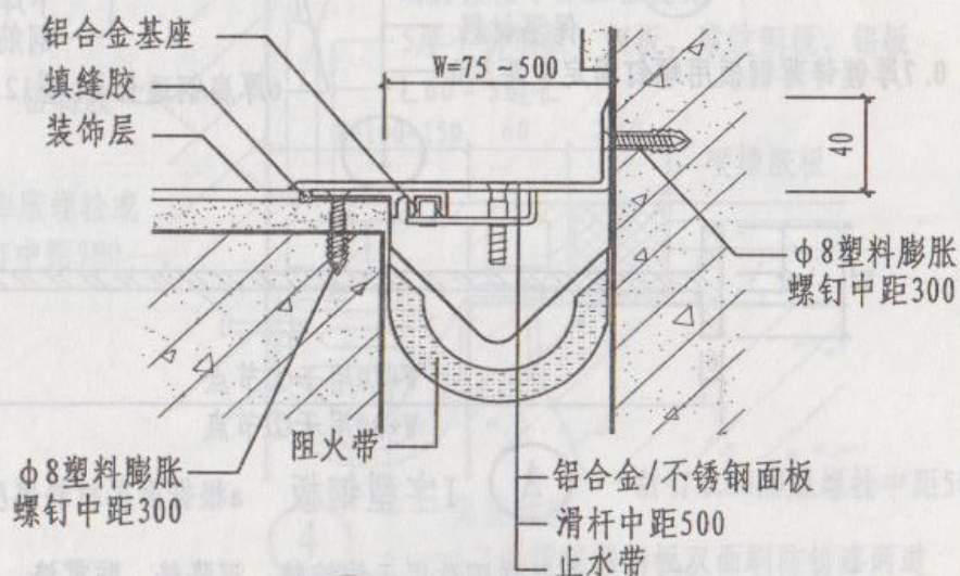
④ 楼、地面与墙面金属盖板型 (后装)
