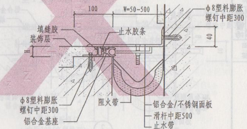
④ 楼、地面与墙面金属盖板胶条型
