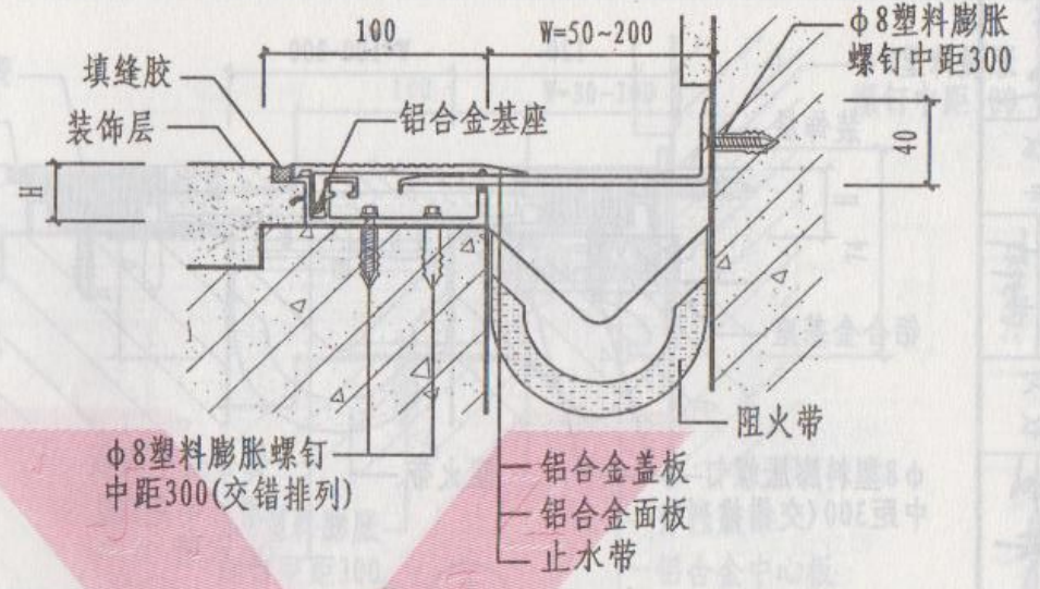
② 楼、地面与墙面金属卡锁型
