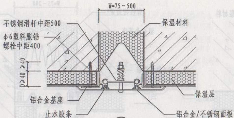
① 外墙盖板防震型
