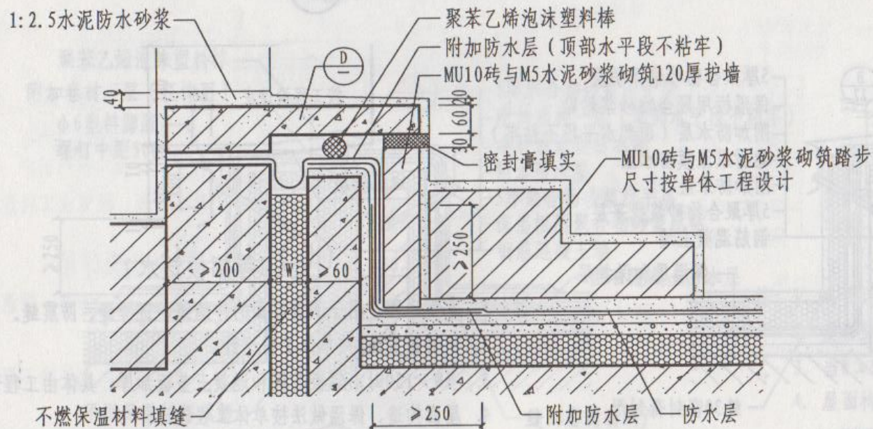
② 屋面出入口变形缝
