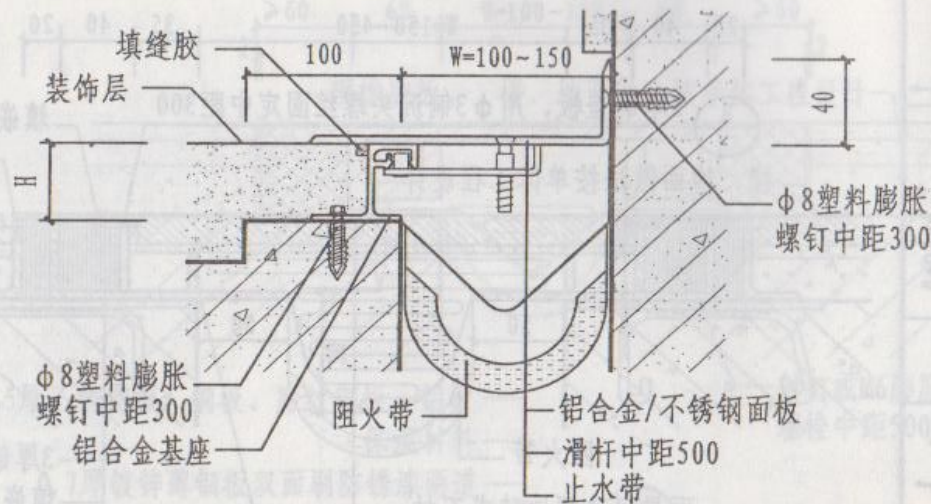
② 楼、地面与墙面金属盖板型
