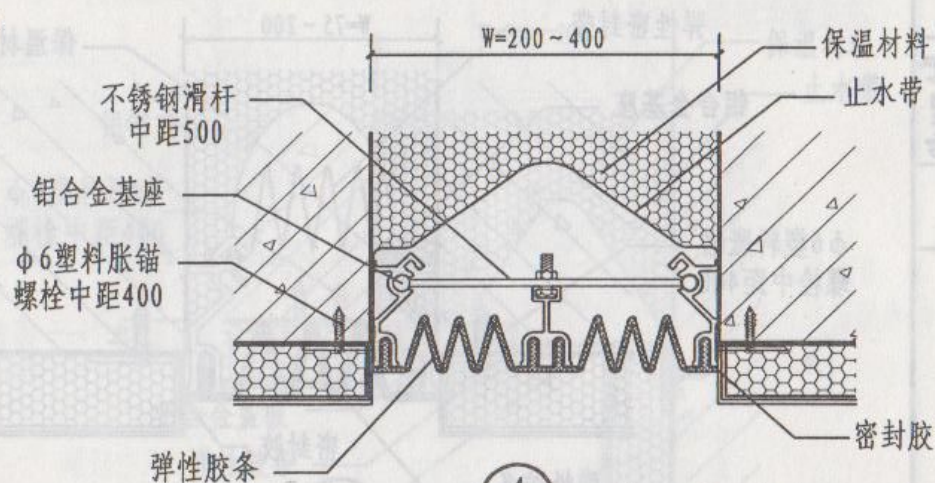
④ 外墙双列胶条防震Ⅱ型
