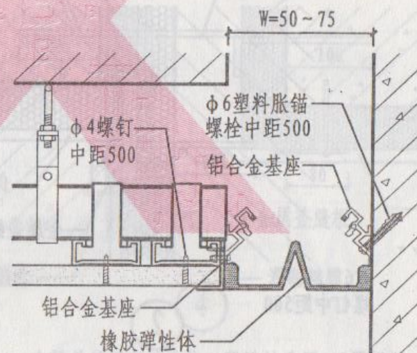
④ 吊顶与内墙橡胶防震 II 型
