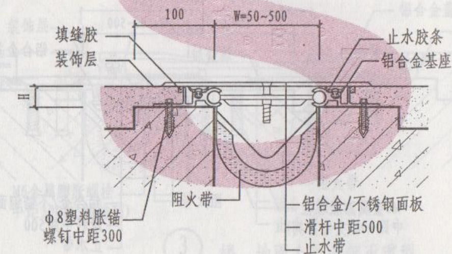
③ 楼、地面金属盖板胶条型
