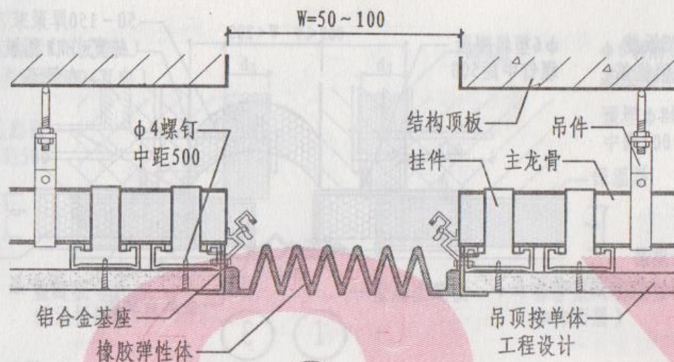
① 吊顶橡胶防震 I 型
