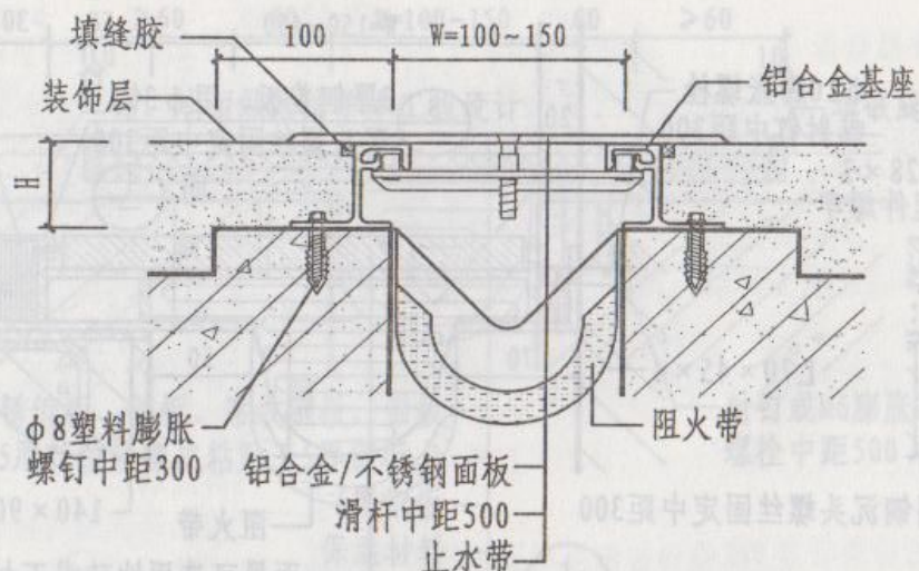
① 楼、地面金属盖板型
