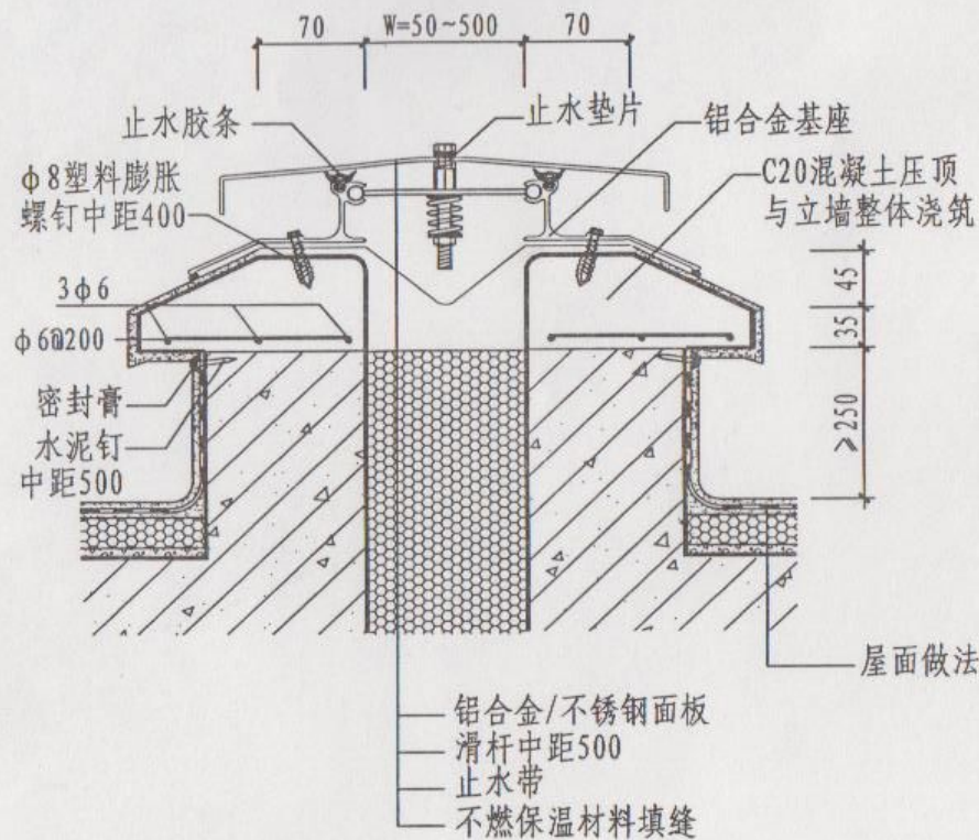
① 屋面金属盖板防震型
