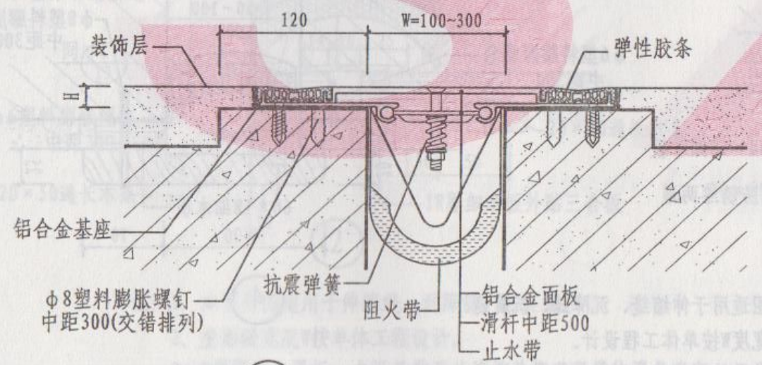
③ 楼、地面双列胶条防震型
