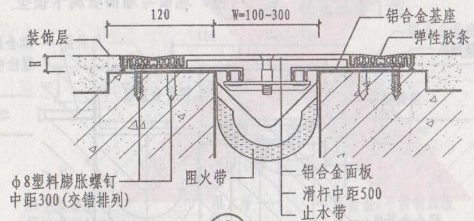
③ 楼、地面双列嵌平胶条型
