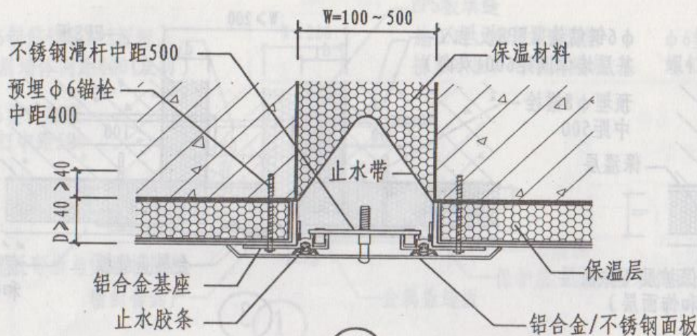
① 外墙金属盖板型
