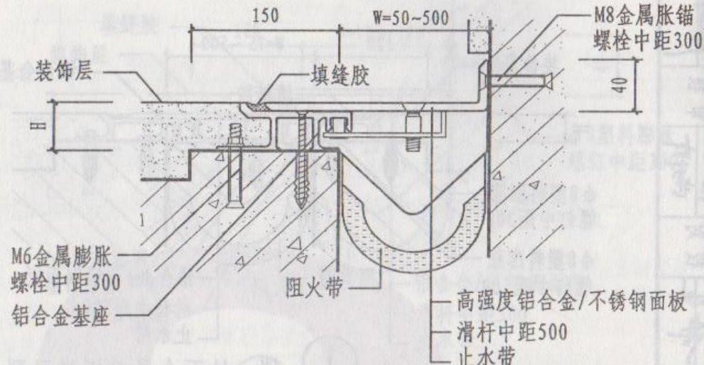
② 楼、地面与墙面承重型
