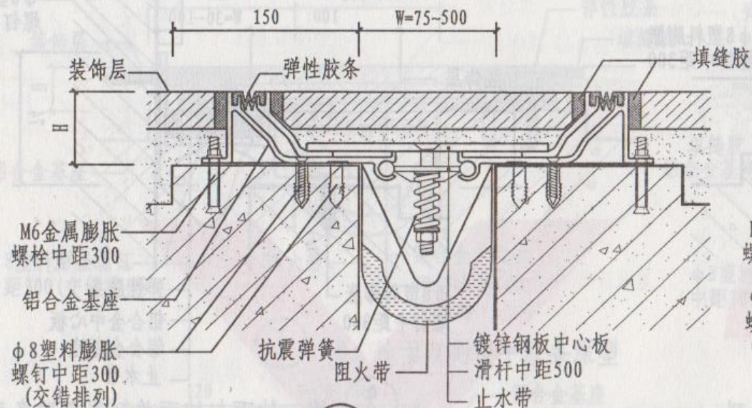
① 楼、地面双列防震型
