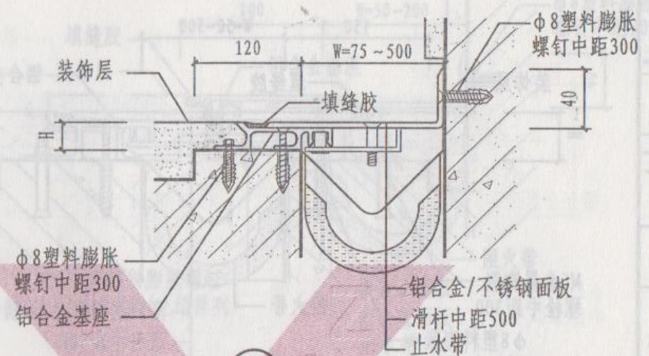
② 楼、地面与墙面金属盖板嵌平型
