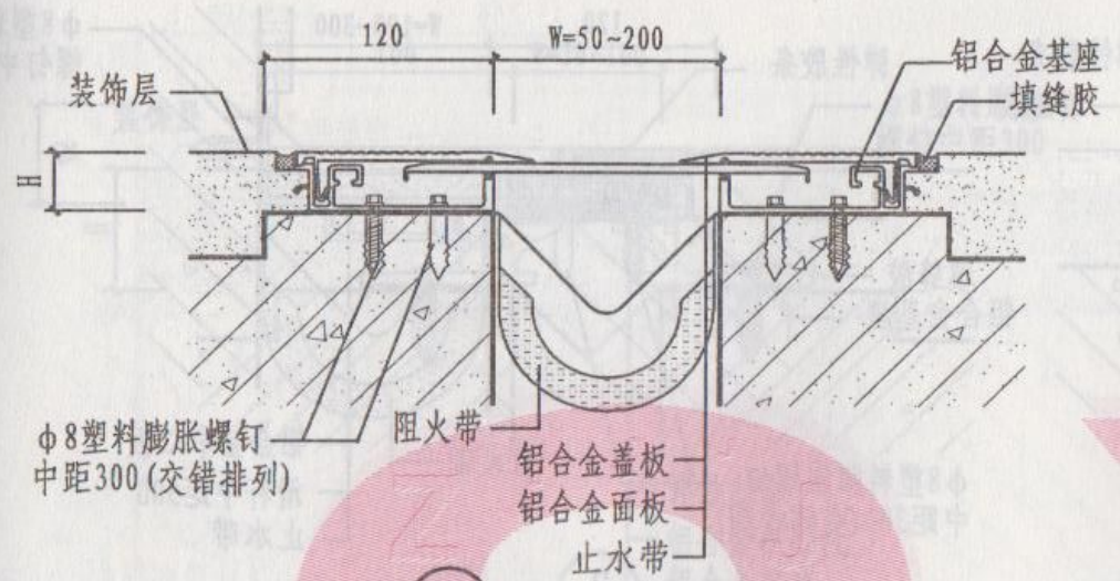
① 楼、地面金属卡锁型
