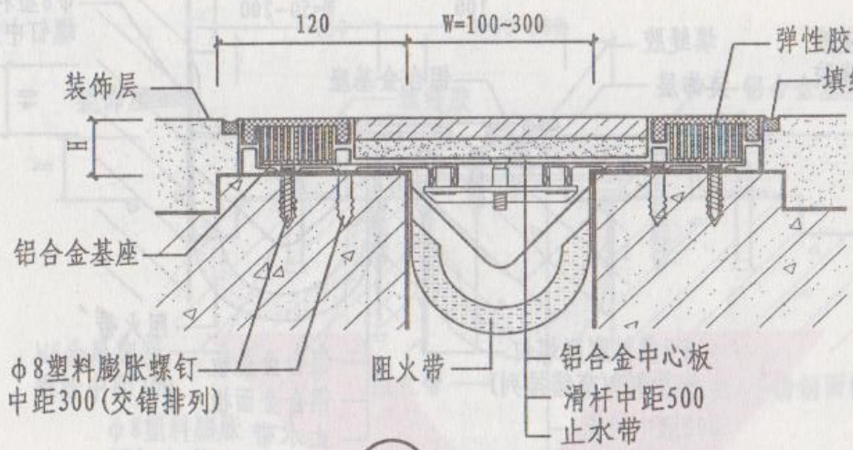
① 楼、地面双列嵌平胶条深型
