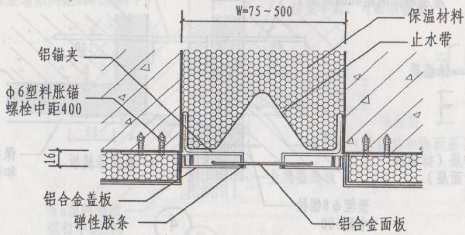
③ 外墙金属卡锁型
