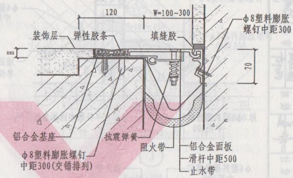
② 楼、地面与墙面双列胶条防震型
