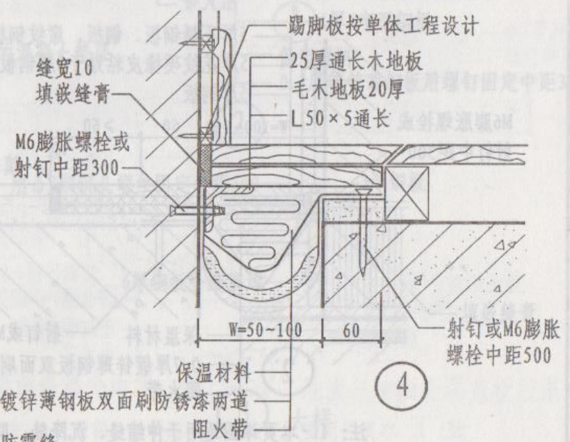
楼、地面变形缝（二）
