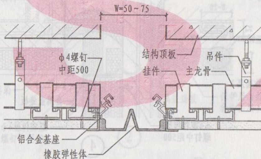
③ 吊顶橡胶防震 II 型
