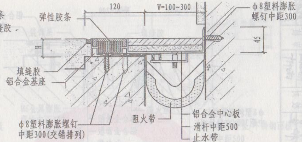
② 楼、地面与墙面双列嵌平胶条深型
