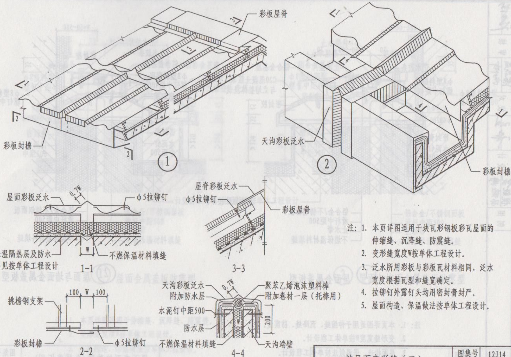
坡屋面变形缝(五)
