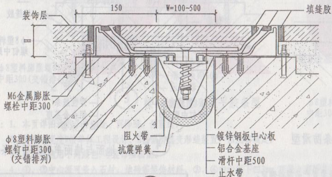
③ 楼、地面胶条防震型
