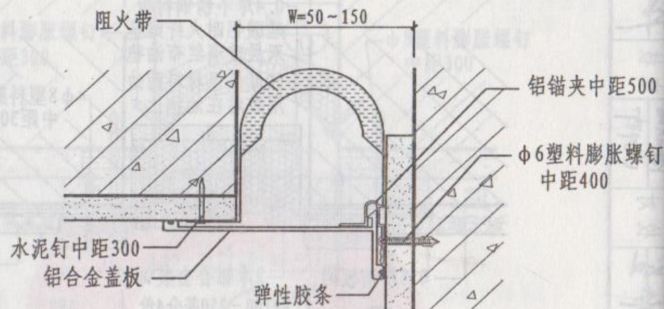
② 内墙、顶棚与内墙单列金属卡锁型
