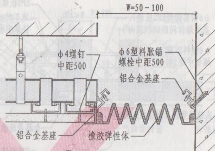
② 吊顶与内墙橡胶防震 I 型
