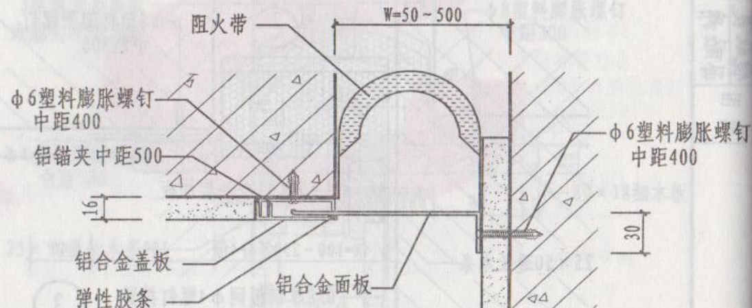
④ 内墙、顶棚与内墙双列金属卡锁型
