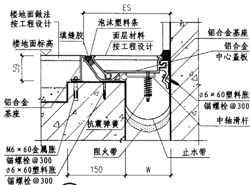
② 楼、地面 (LAP) 转角型
