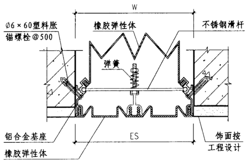
① 外墙 (QTT-1)
