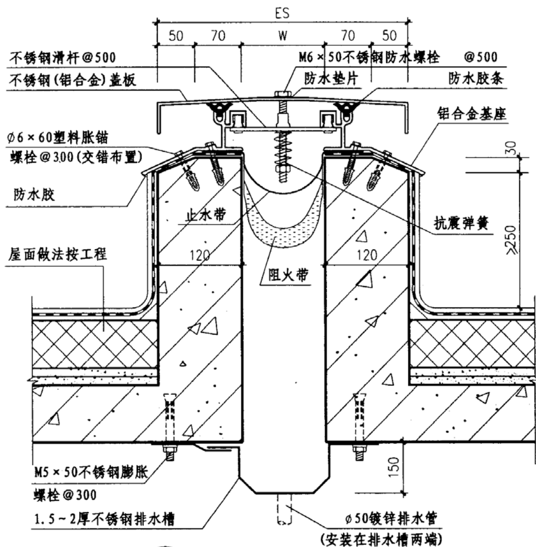
① 屋面变形缝 (QCC-1) 平面型
