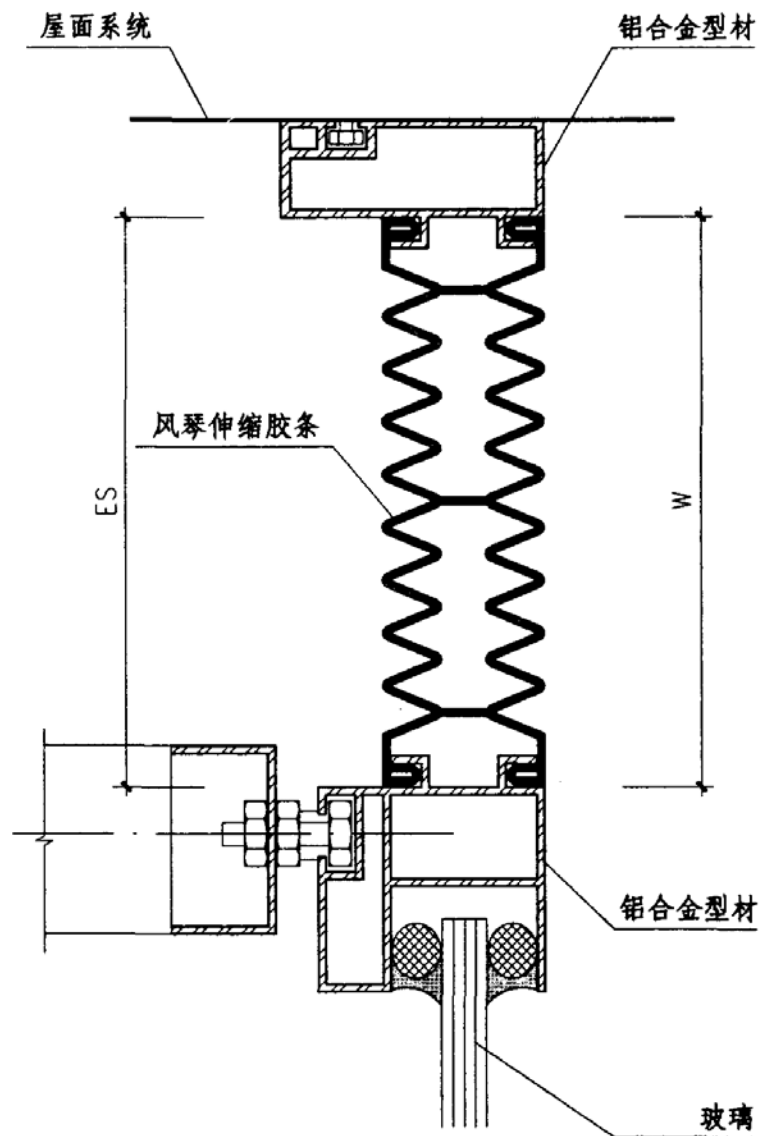
① 棚顶与玻璃之间 (QTTW)
