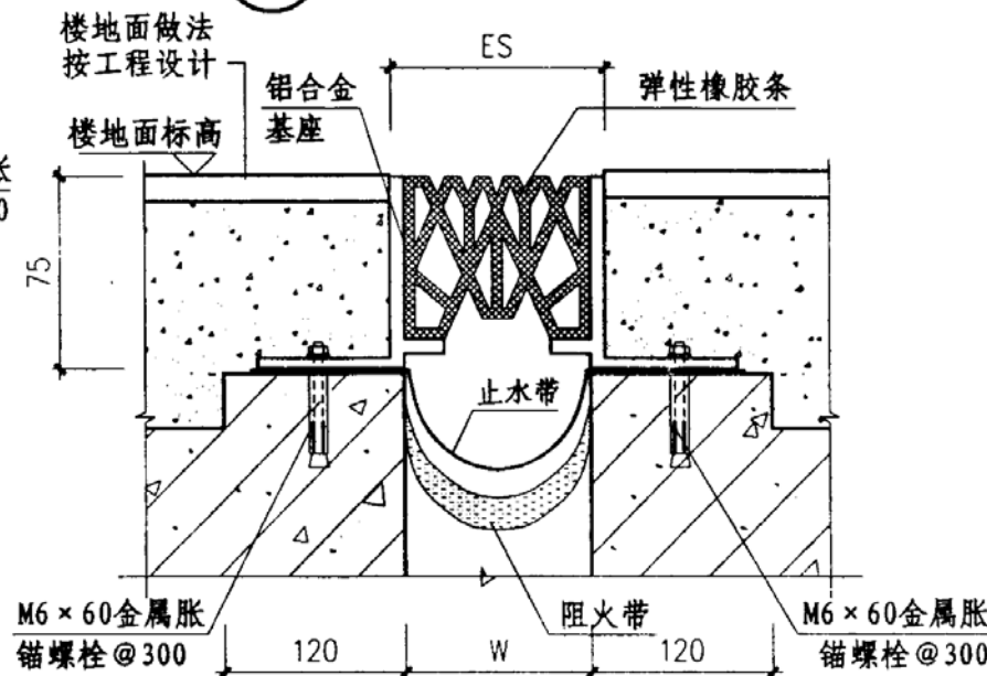
④ 楼、地面 (QTP) 平面型
