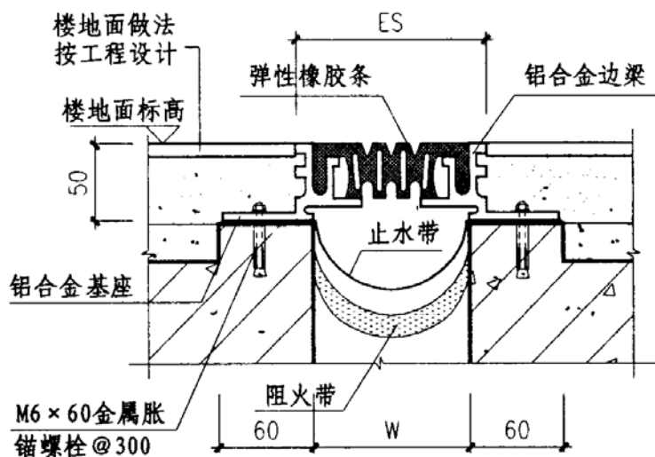
③ 楼、地面 (QFA) 平面型
