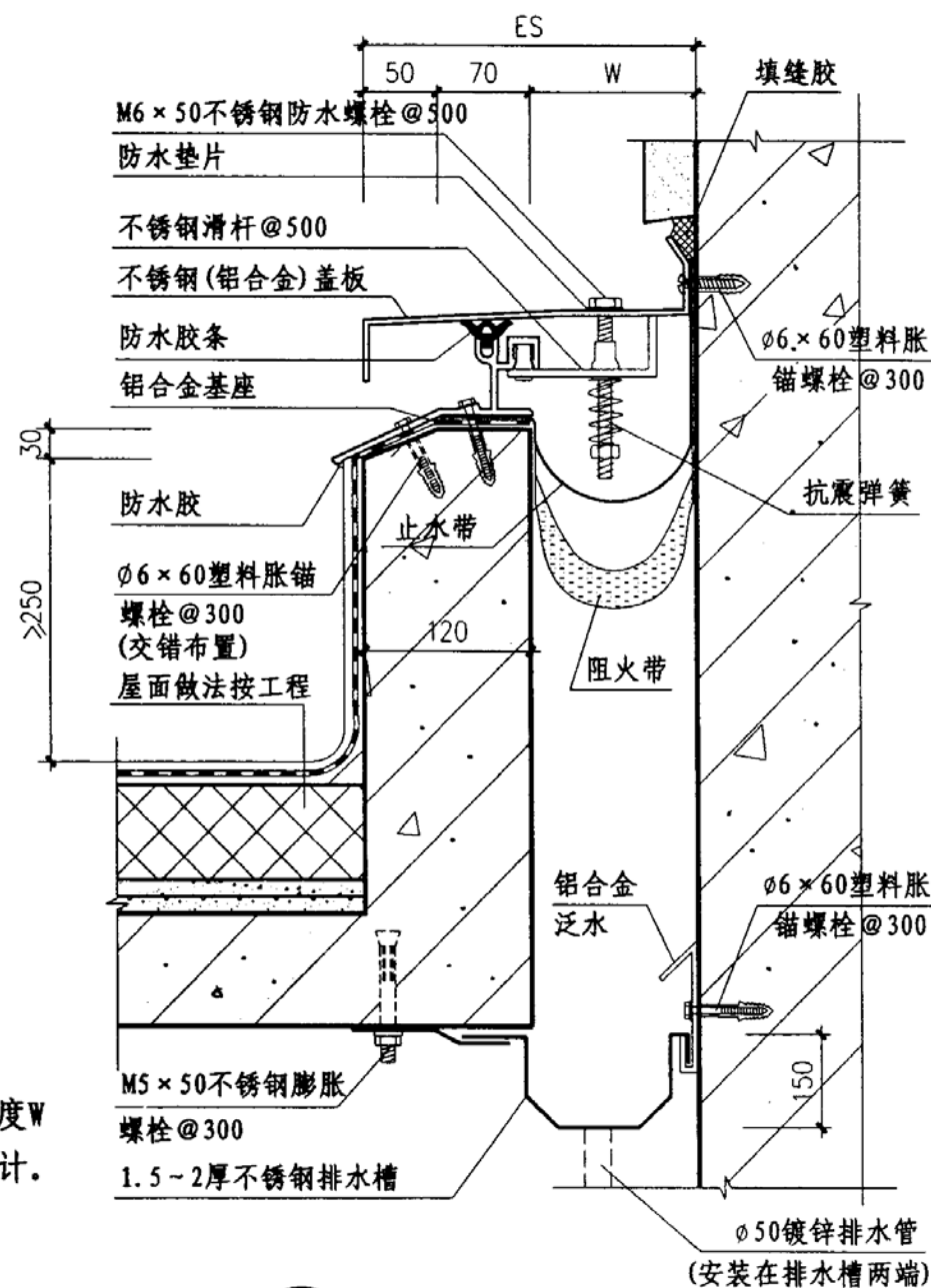
② 屋面变形缝 (LCC-1) 转角型
