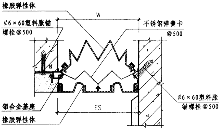
④ 外墙 (LTT-2)
