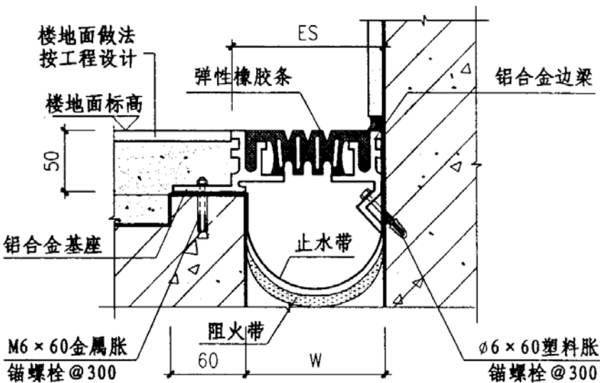
④ 楼、地面 (LFA) 转角型
