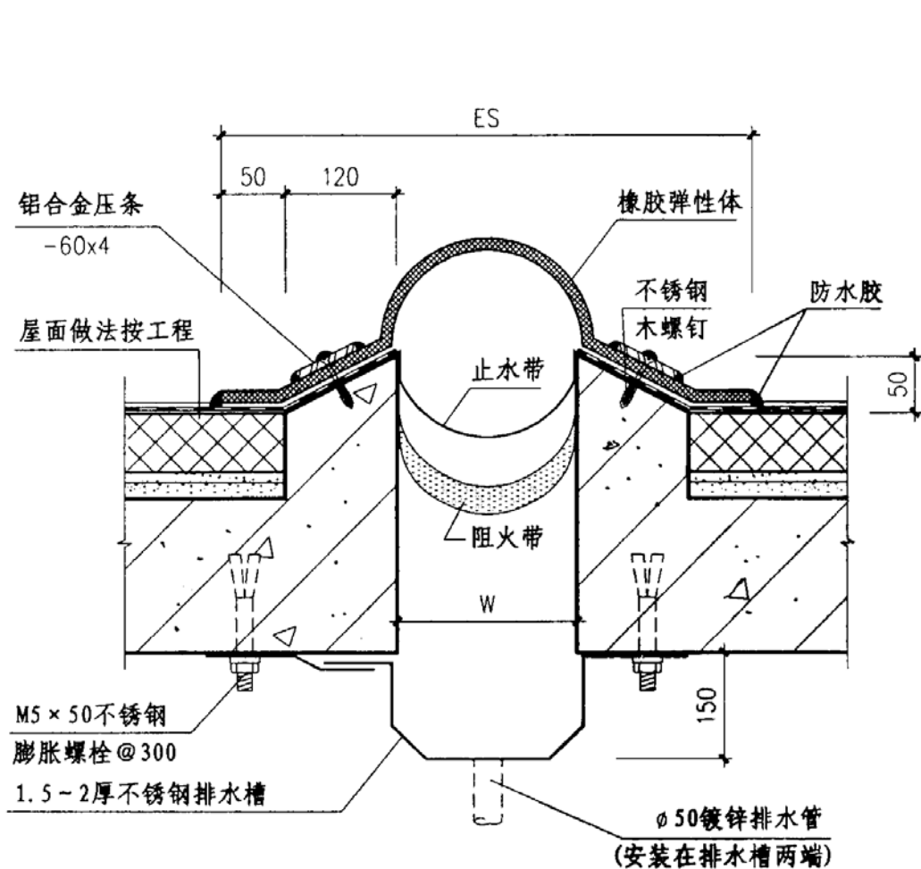
① 屋面变形缝 (QTTL) 平面型
