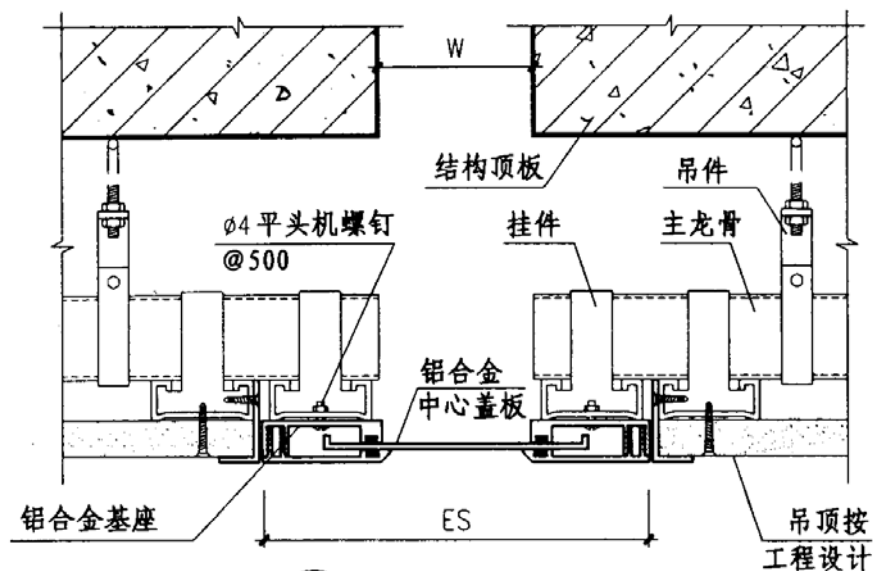
① 吊顶 (QAD)
