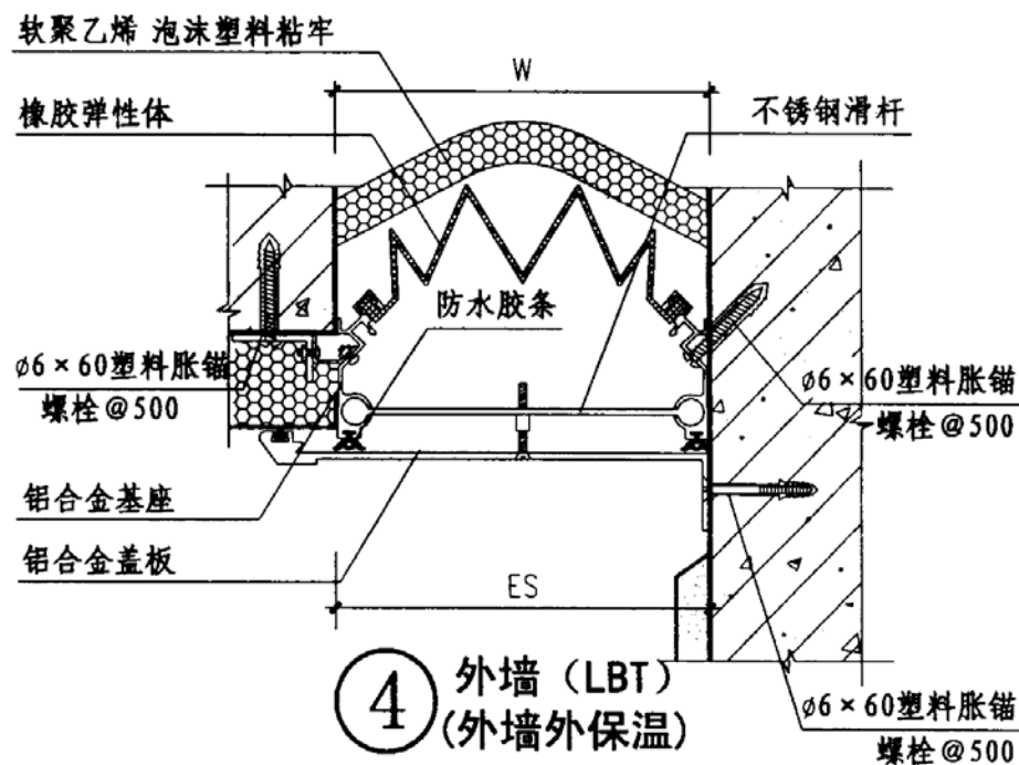
金属盖板型外墙变形缝
