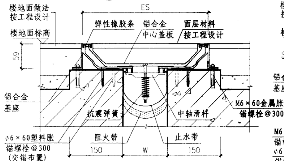
③ 楼、地面 (QAH) 平面型
