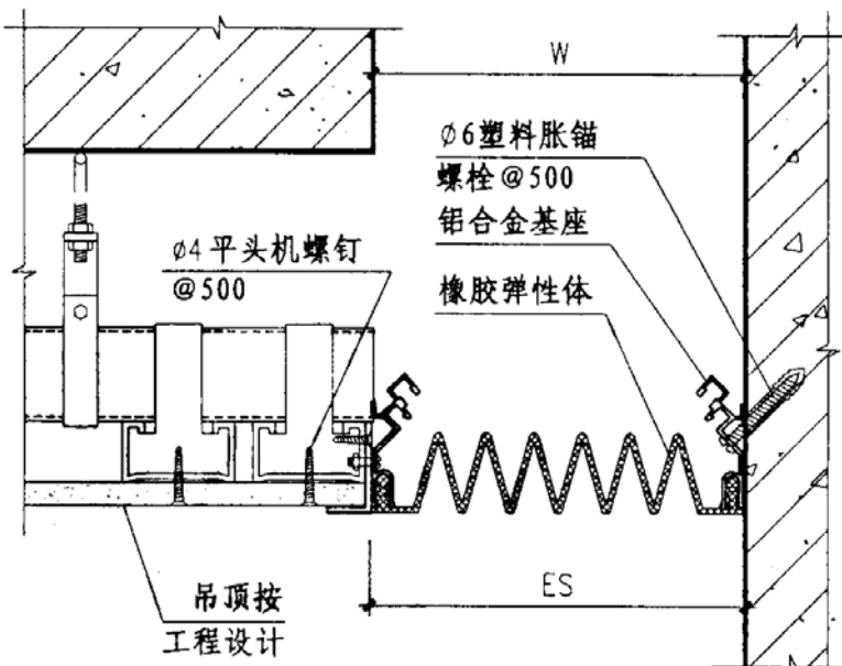
② 吊顶 (LTT-1)
