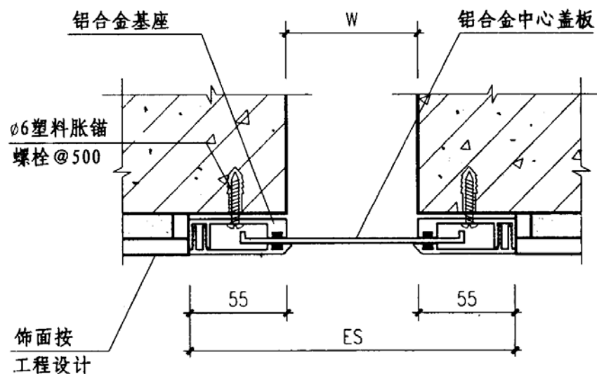
③ 墙面、顶棚 (QAD)
