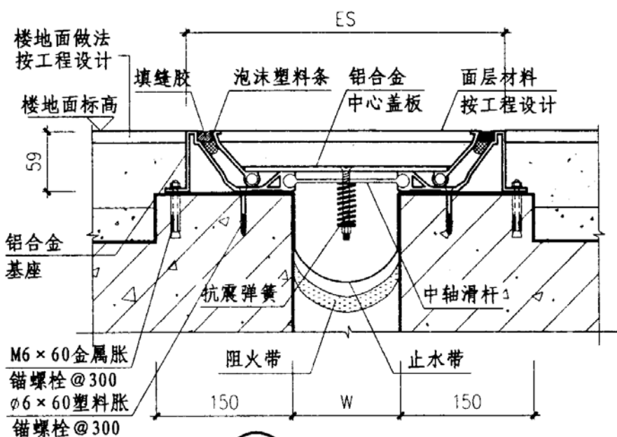
① 楼、地面 (QAP) 平面型
