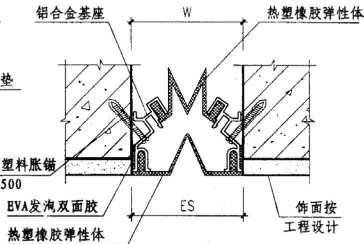
② 外墙 (QTT-4)
