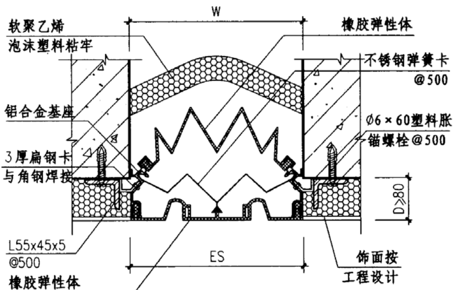
③ 外墙 (QTT-2) (外墙外保温)
