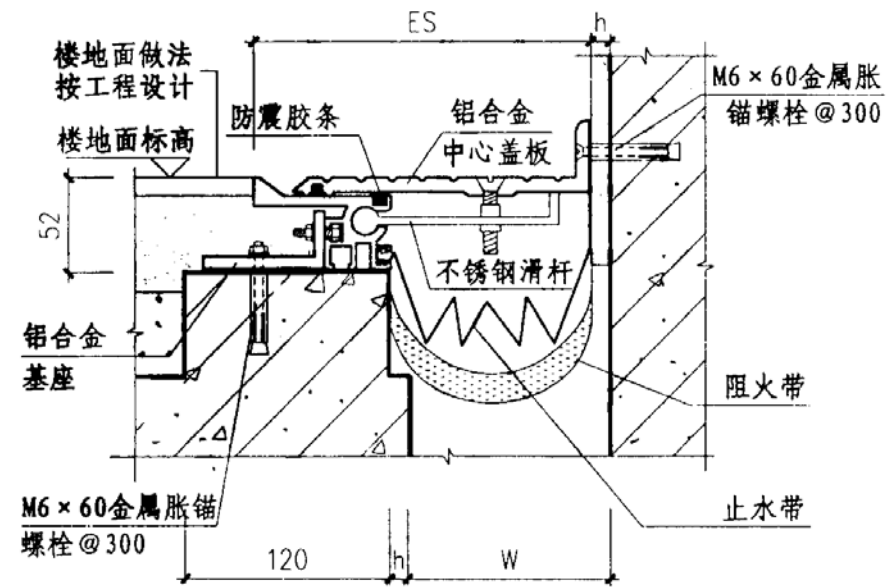
④ 楼、地面 (LAHD) 转角型
