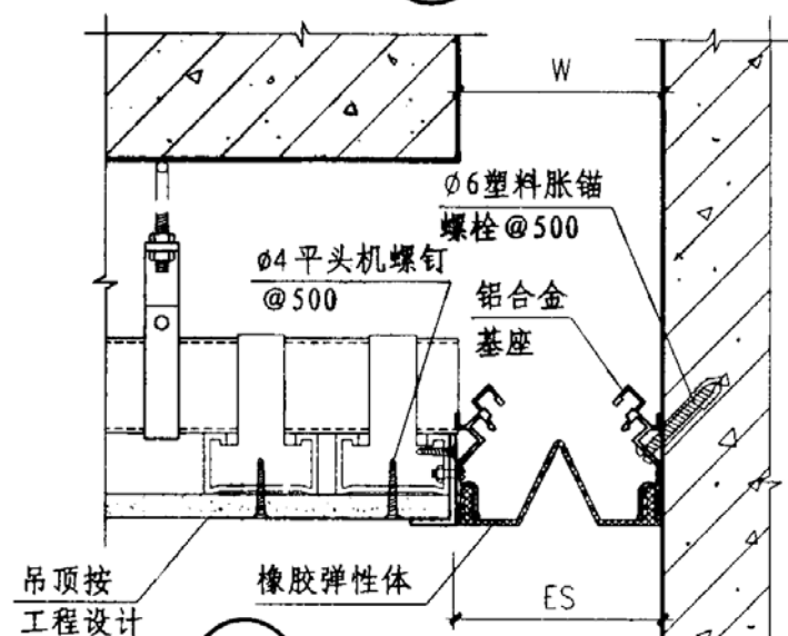
④ 吊顶 (LTT-2)
