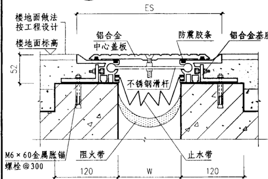
③ 楼、地面 (QAHD) 平面型
