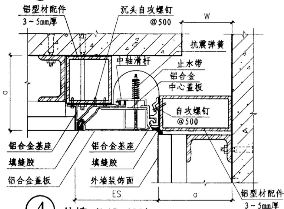
② 外墙 (LBH-400)
