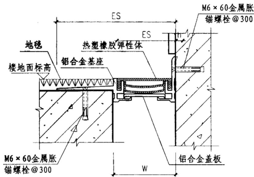
④ 楼地面 (LT0) 转角型
