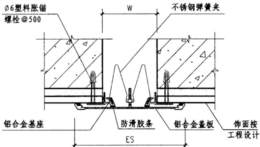
① 墙面、顶棚 (QFAH)
