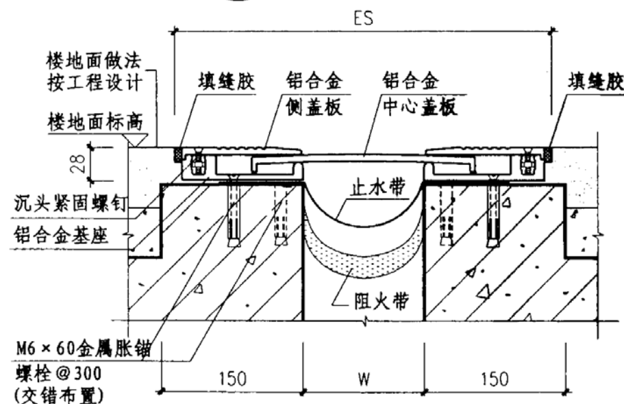
③ 楼、地面 (QADU) 平面型
