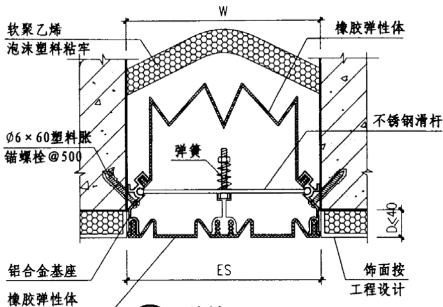
① 外墙 (QTT-1) (外墙外保温)
