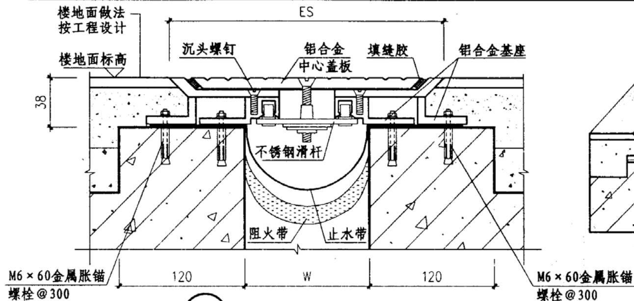
① 楼、地面 (QAAH) 平面型
