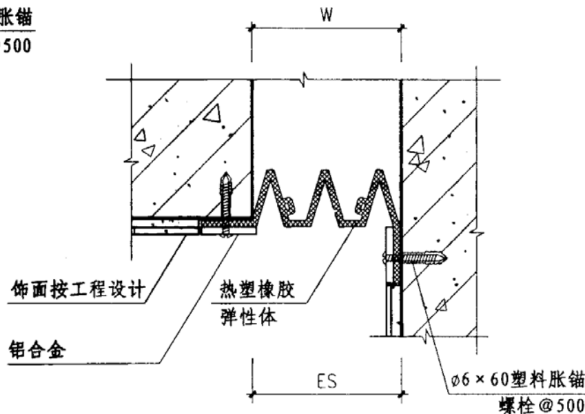
④ 外墙 (LFAX)
