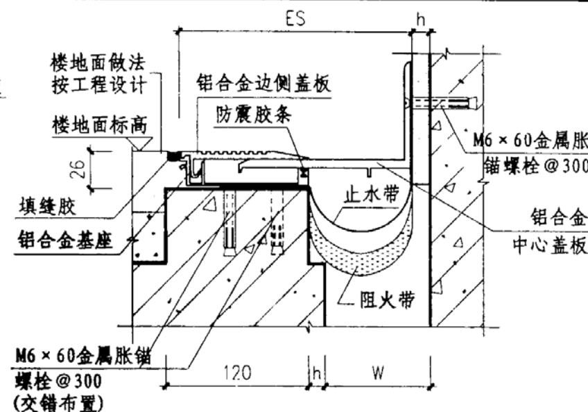
② 楼、地面 (LAHR) 转角型
