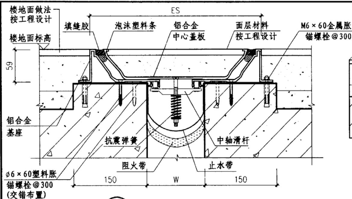
① 楼、地面 (QAA) 平面型
