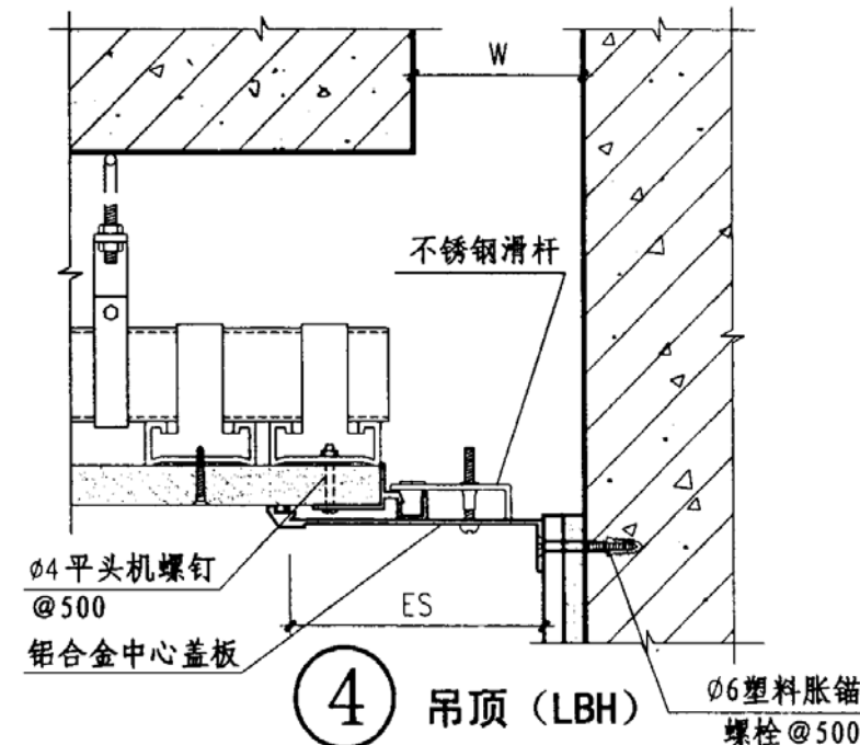
② 吊顶 (LAD)
