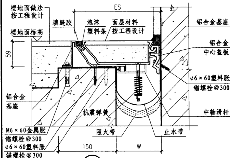
② 楼、地面 (LAA) 转角型
