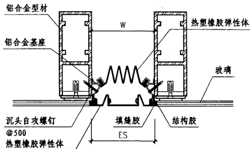
③ 玻璃外墙 (QTT-3)
