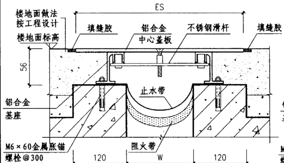
③ 楼、地面 (QBC) 平面型
