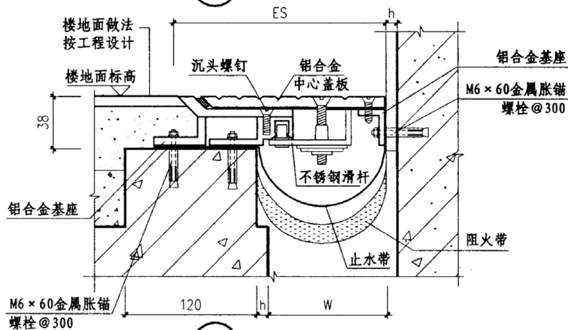
② 楼、地面 (LAAH) 转角型
