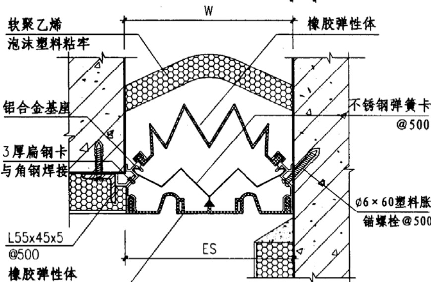
④ 外墙 (LTT-2) (外墙外保温)
