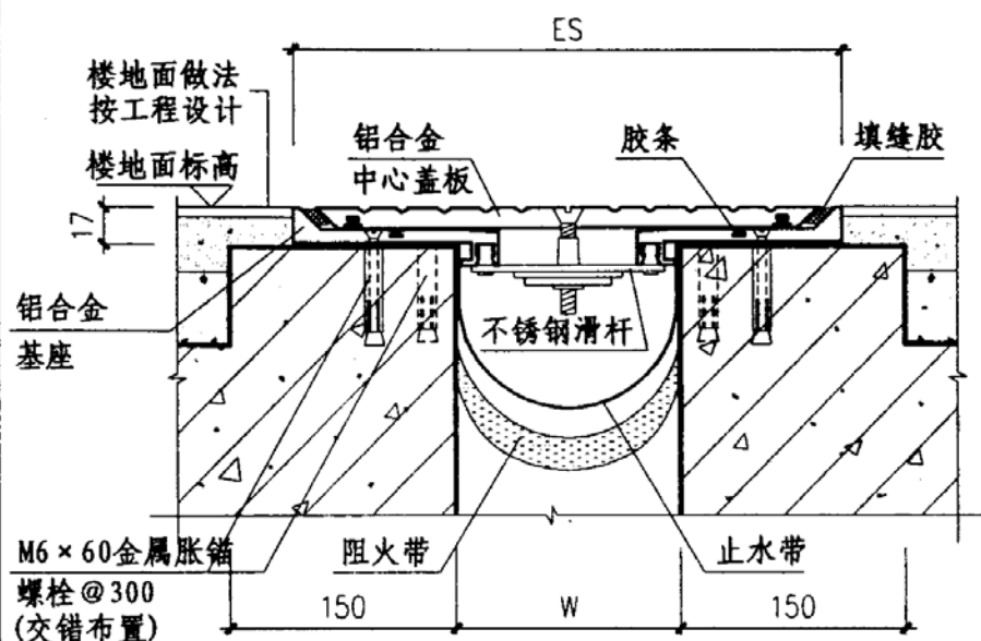
① 楼、地面 (QAHP) 平面型
