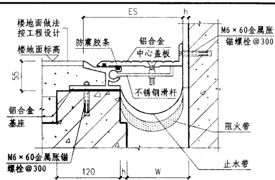
② 楼、地面 (LAHH) 转角型
