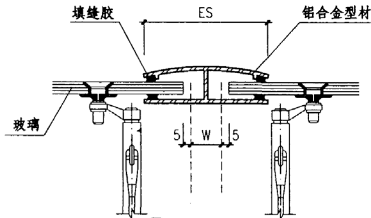
② 玻璃外墙 (QPP)
