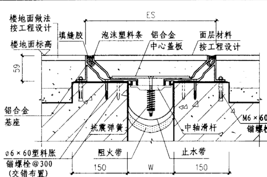
① 楼、地面 (QAB) 平面型
