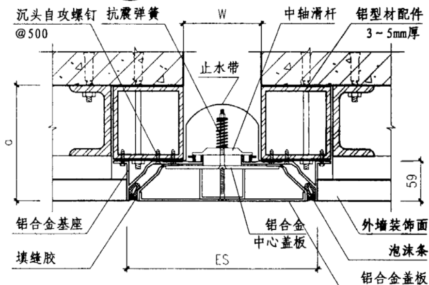
③ 外墙 (QAB-400)
