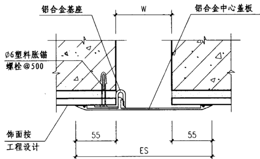
① 墙面、顶棚 (QADR)
