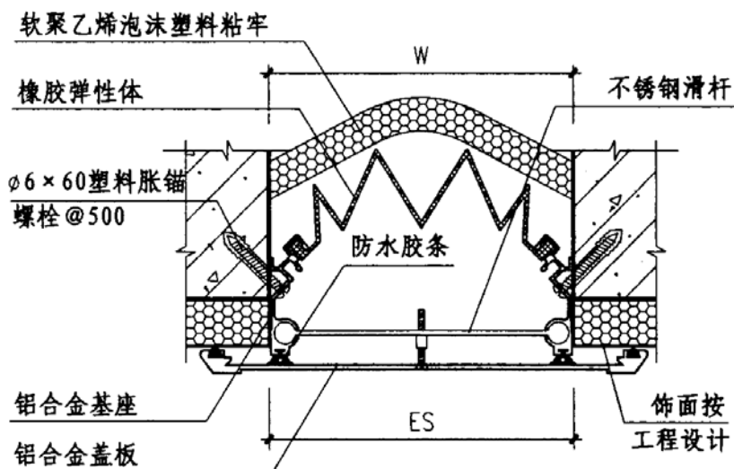
③ 外墙 (QBT) (外墙外保温)
