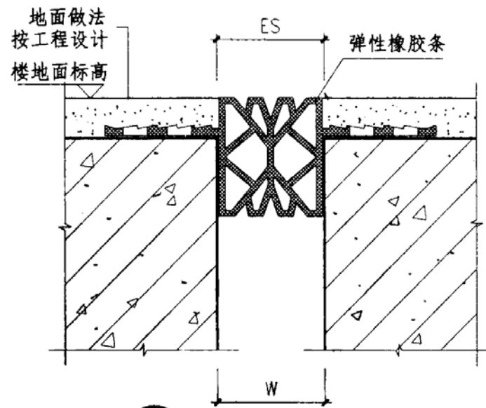
② 楼地面 (TPT-1) 平面型
