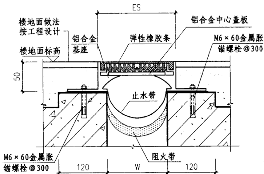
③ 楼、地面 (QFAG) 平面型
