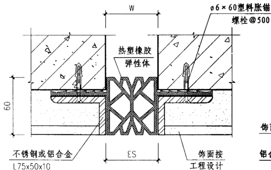
③ 外墙 (QTF)
