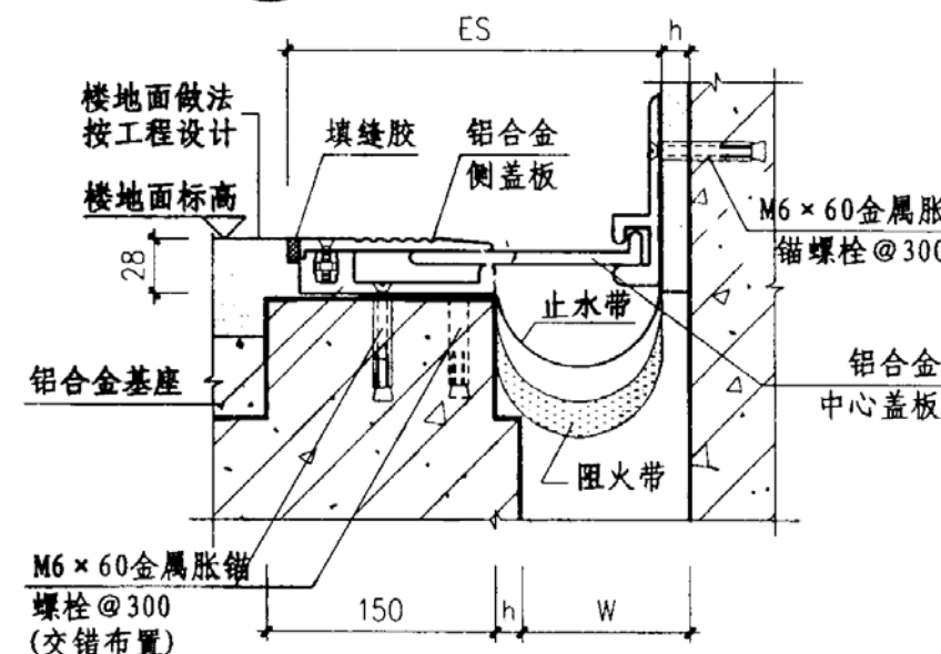
④ 楼、地面 (LADU) 转角型
