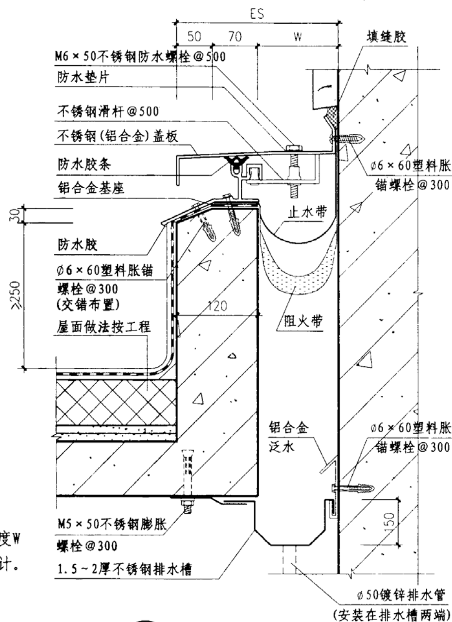
② 屋面变形缝 (LCC) 转角型
