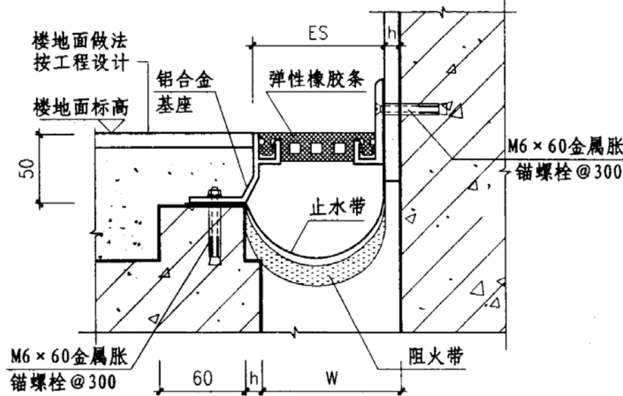
② 楼、地面 (LFAJ) 转角型
