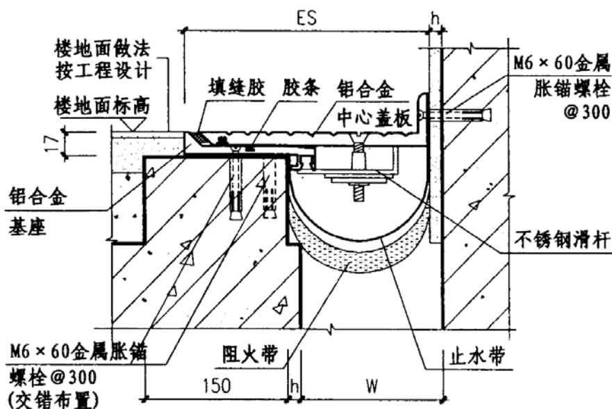
② 楼、地面 (LAHP) 转角型
