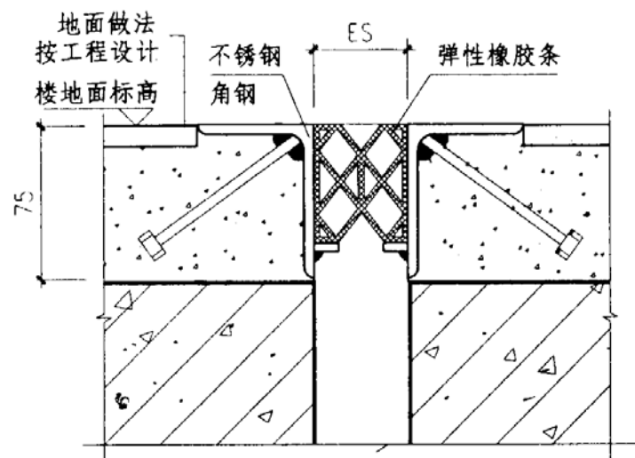
① 楼地面 (QPP) 承重型
