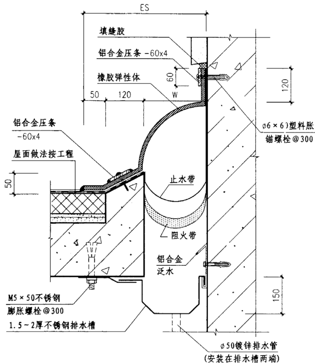
② 屋面变形缝 (LTTL) 转角型
