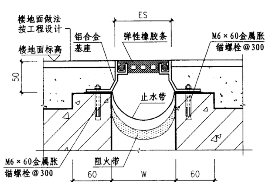
① 楼、地面 (QFAJ) 平面型
