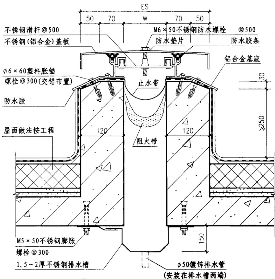
① 屋面变形缝 (QCC) 平面型
