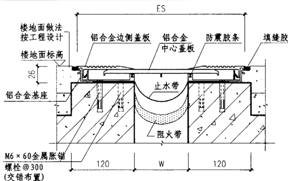
① 楼、地面 (QAHR) 平面型
